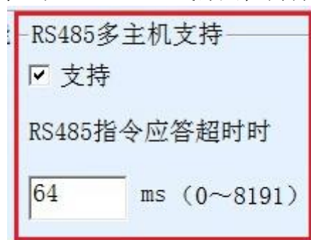
图 37 RS485 多主机支持
