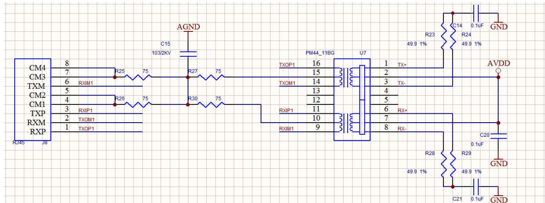
图 9 RJ45 和网络变压器分开方式
