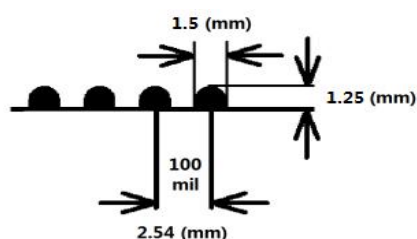
图 5 ZLSN2003T 邮票孔尺寸
