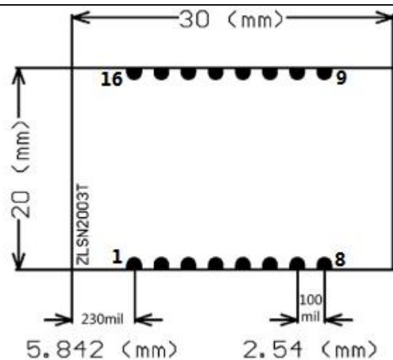
图 4 ZLSN2003T 正面引脚图
