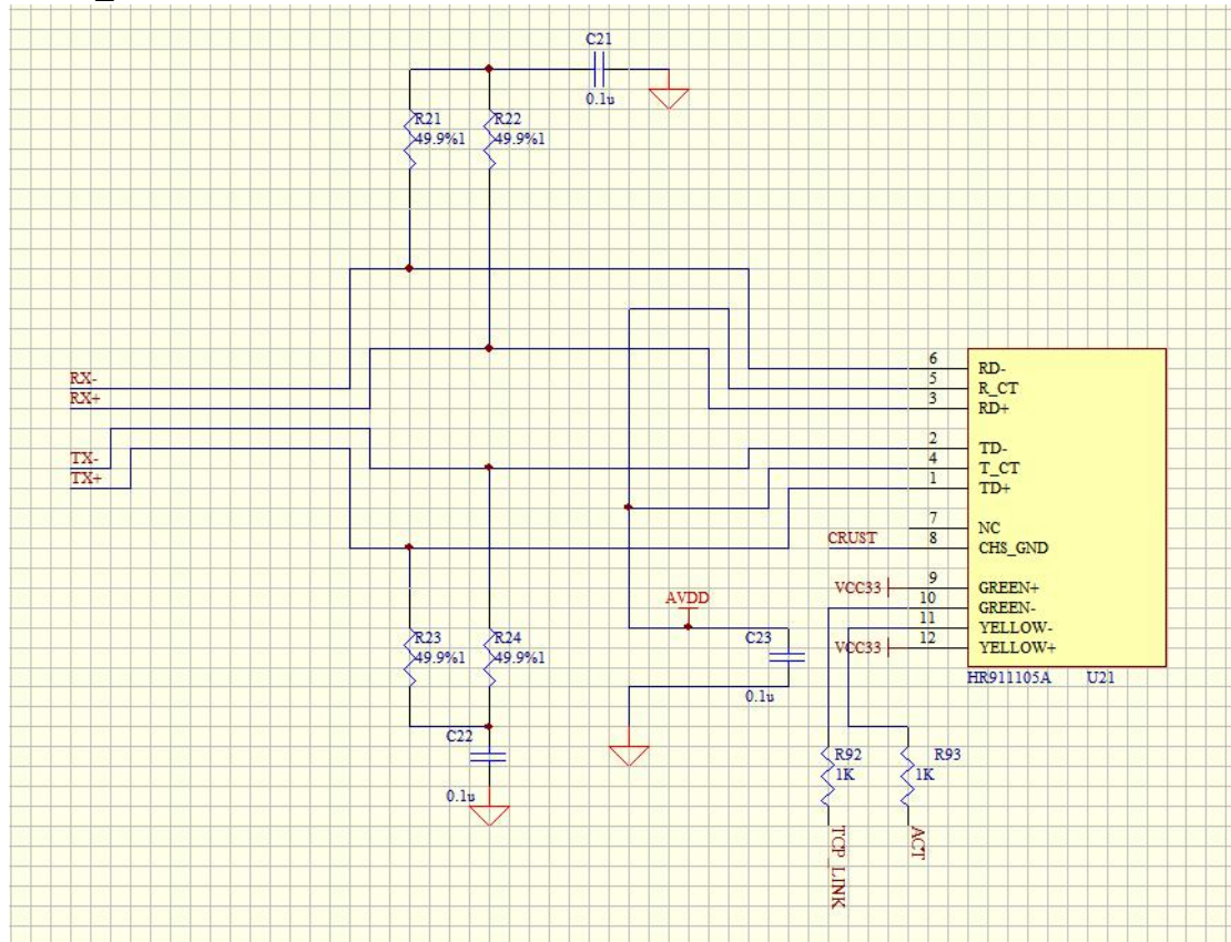
图 8 带网络变压器 RJ45
