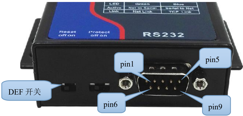
图 5 RS232 接口和拨码
