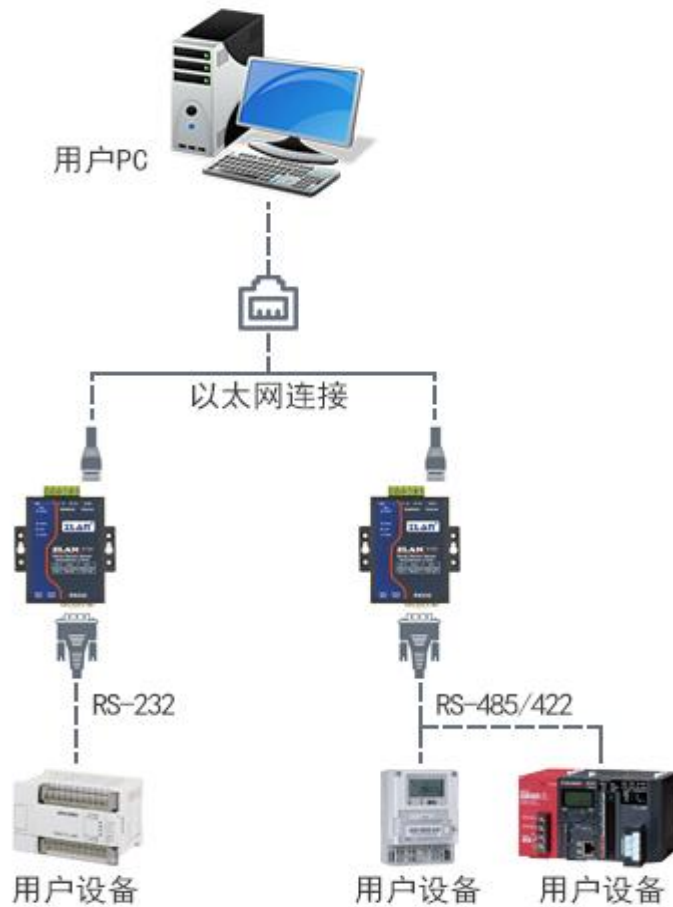
图 2 连接示意图
