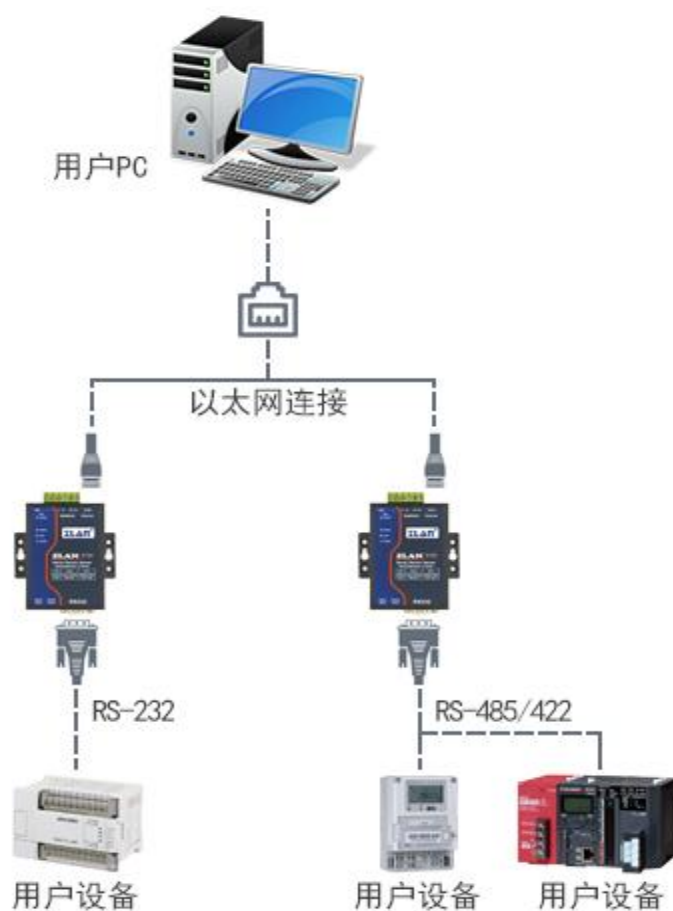
图 2 连接示意图
