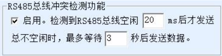
图 39 RS485 防冲突空闲时间
