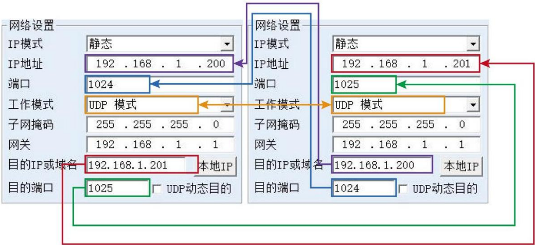
图 29 UDP 设备对联参数配置
