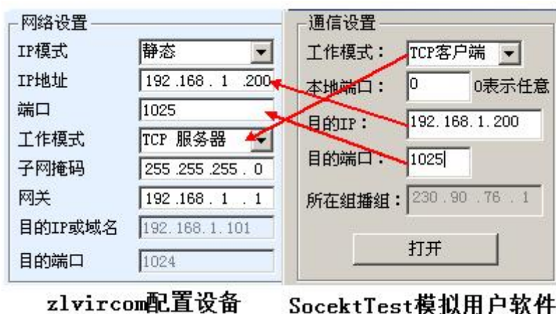
图 24 串口服务器作为服务端
