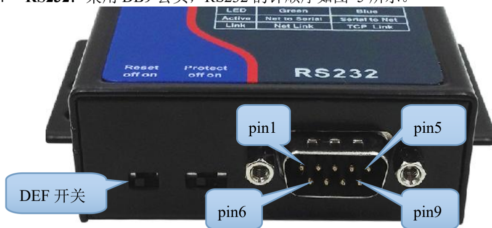
图 5 RS232 接口和拔码
