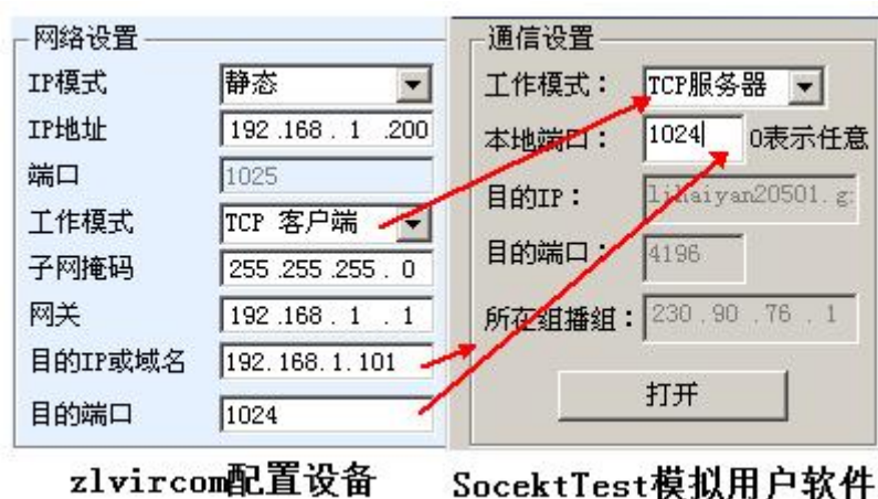
图 20 串口服务器作为客户端
