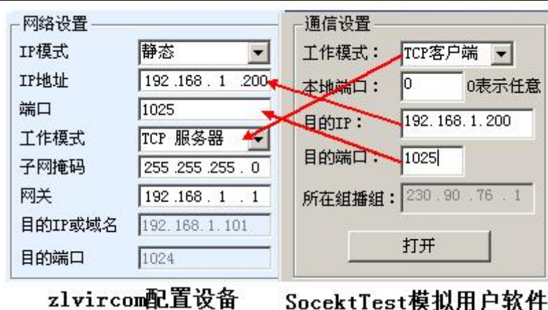
图 23 串口服务器作为服务端
