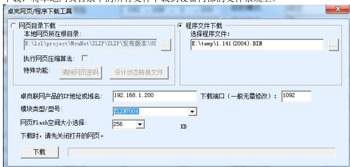
图 51 ZLAN2003 web 升级方法
