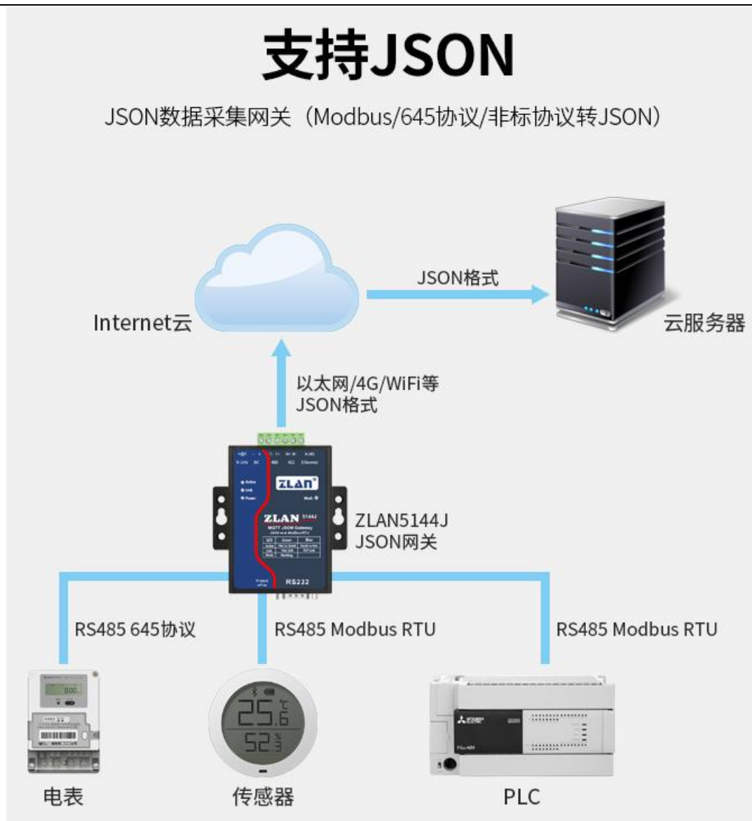
图 2 ZLAN5144 网络结构
