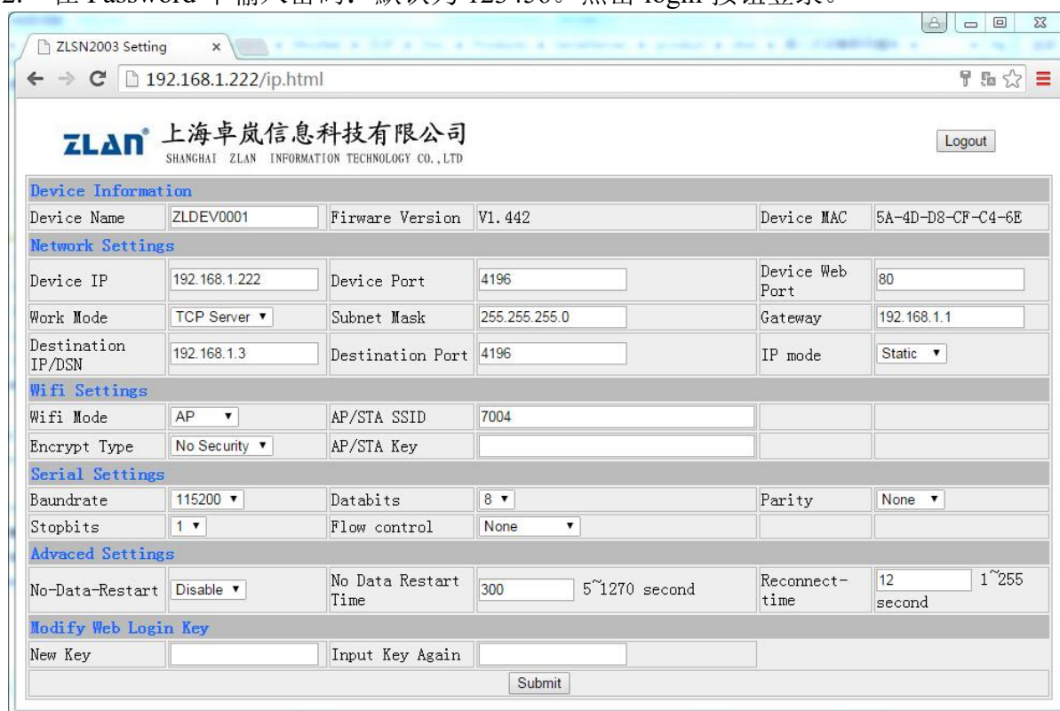
图 19 Web 配置界面
