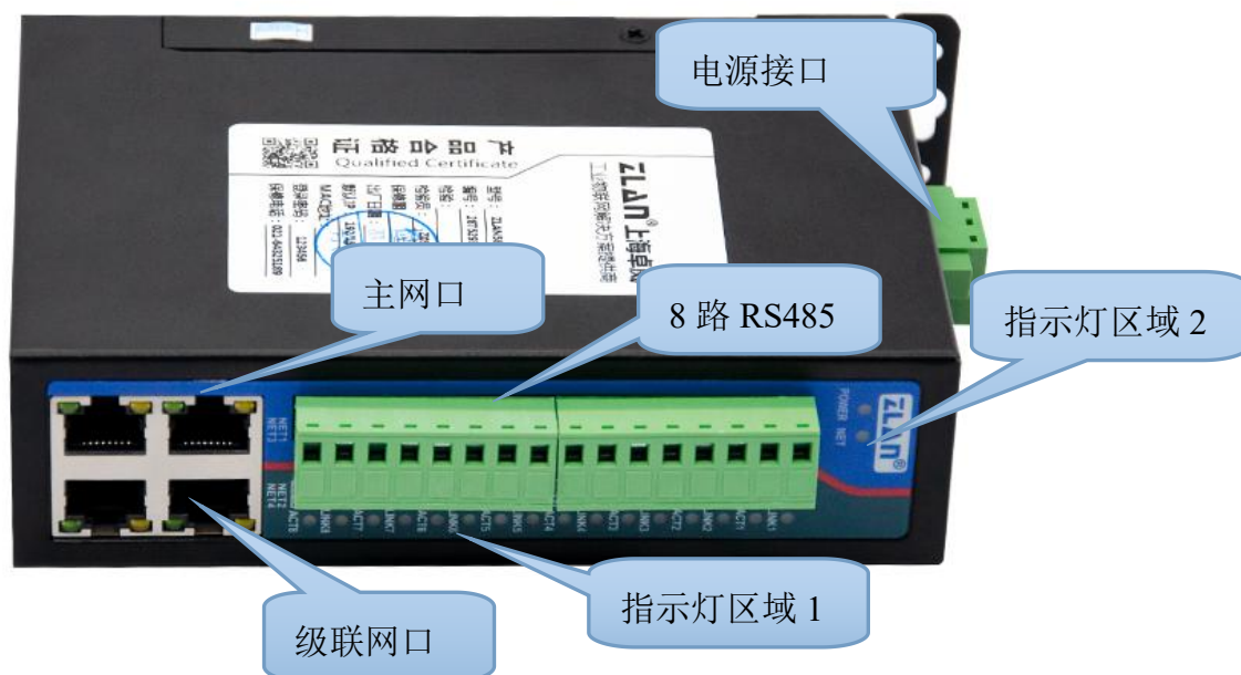
图 3 正视图
