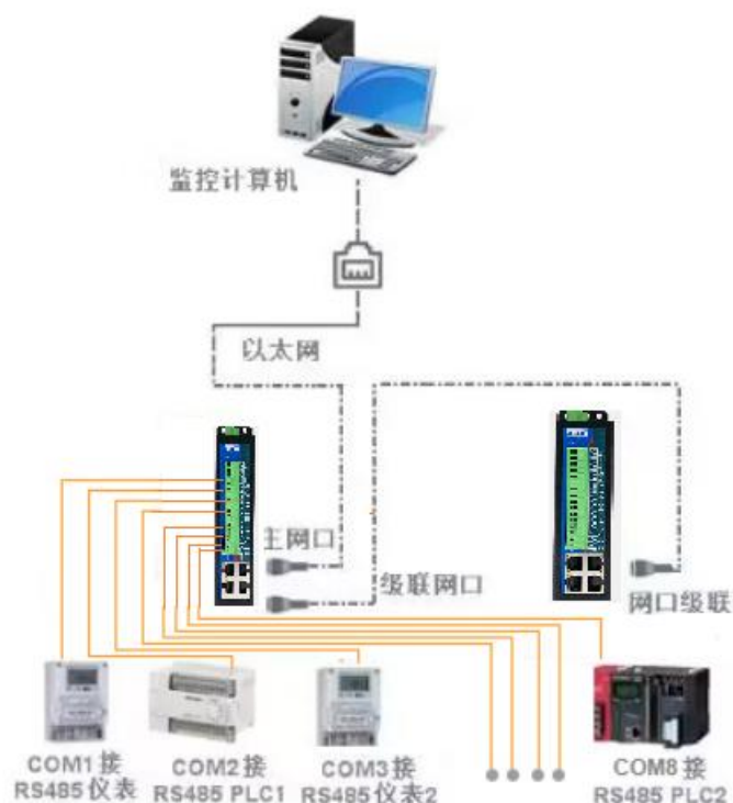
图 2 连接示意图
