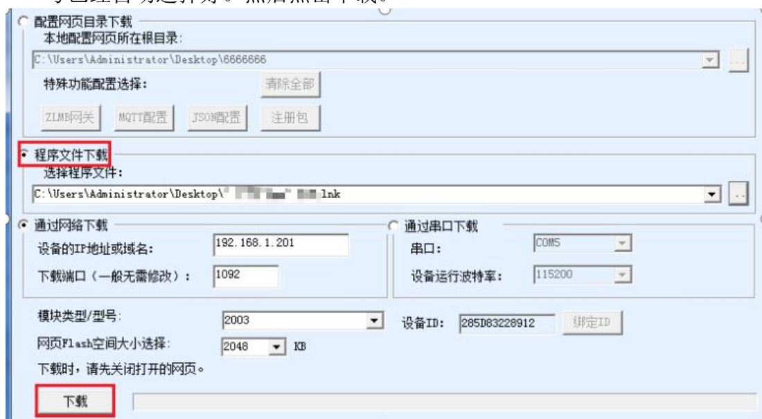
图 59 ZLAN5812D 固件升级方法
