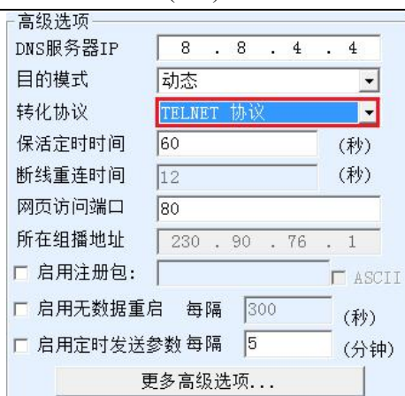
图 32 TELNET 协议
