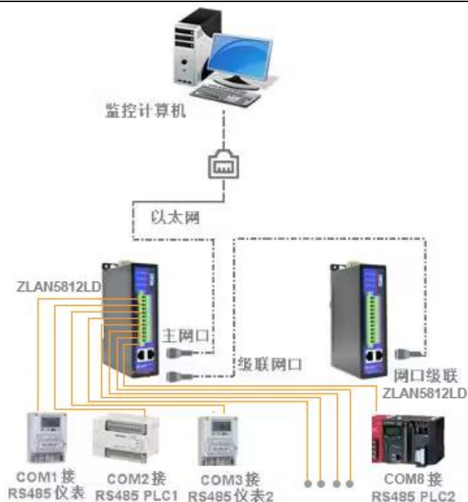
图 2 连接示意图
