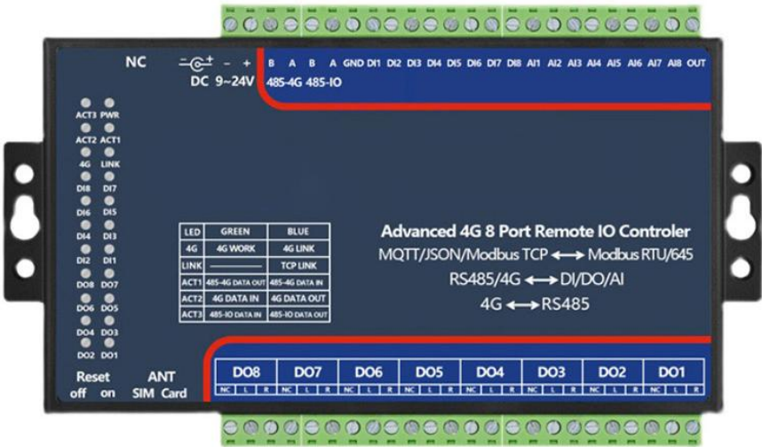
图 4 ZLAN6808I-8
