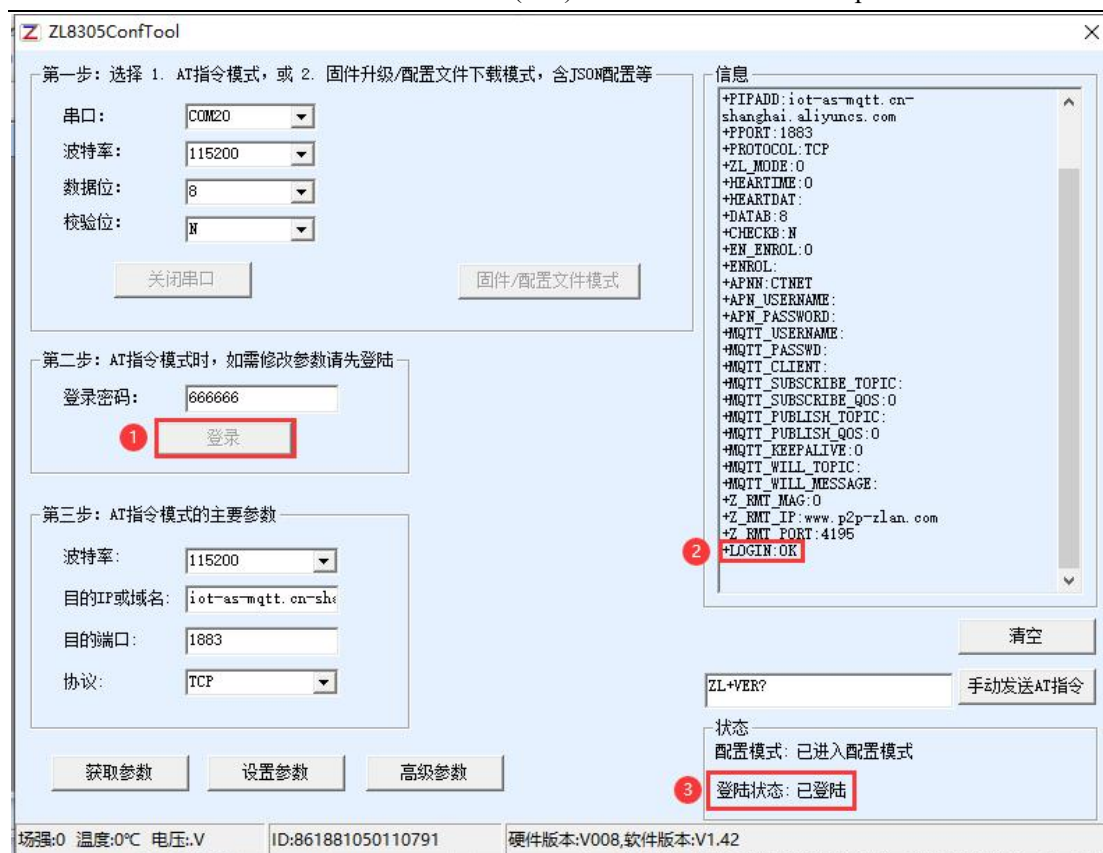
图 32 登录页面
