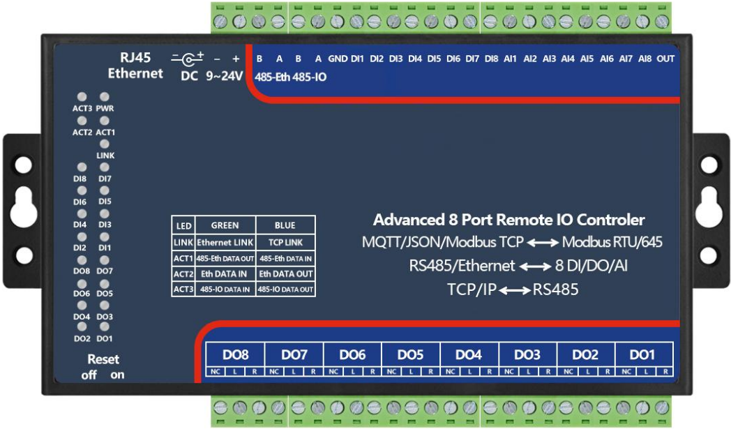
图 2 ZLAN6808I-8 正面图
