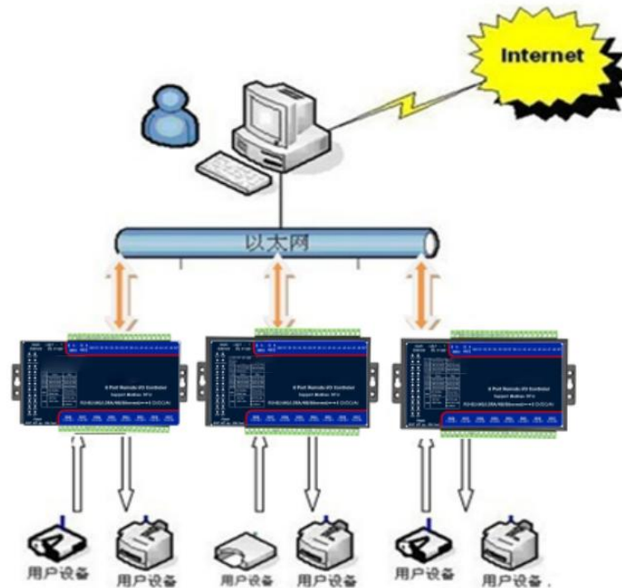
图 3 连接案例
