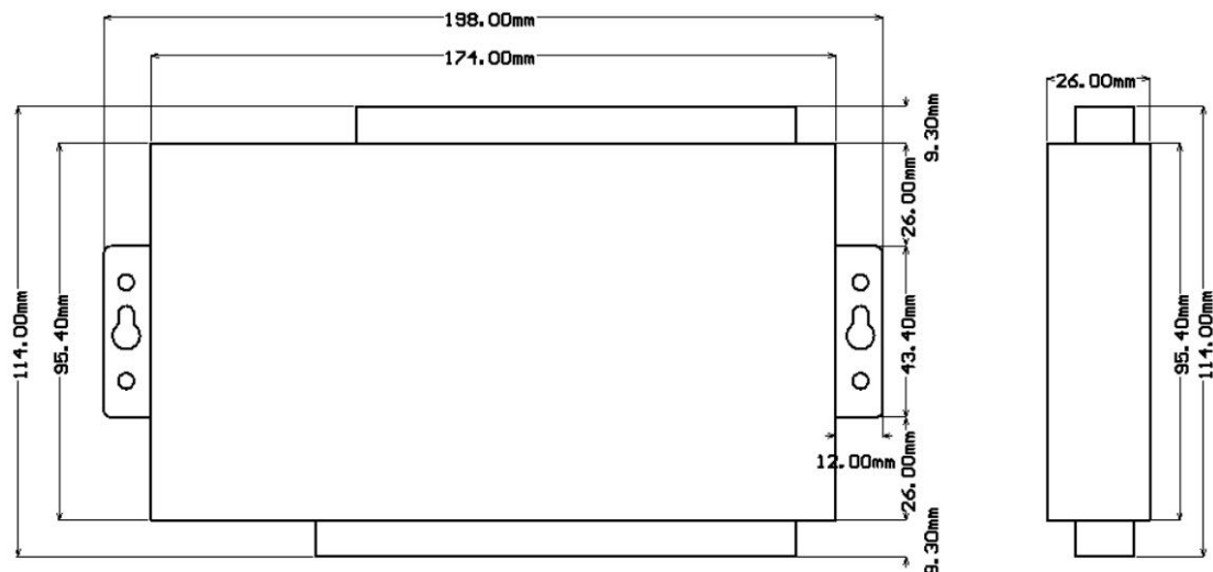
图 586808I 尺寸图
