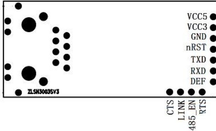
图 3 ZLSN3003S pin 脚
