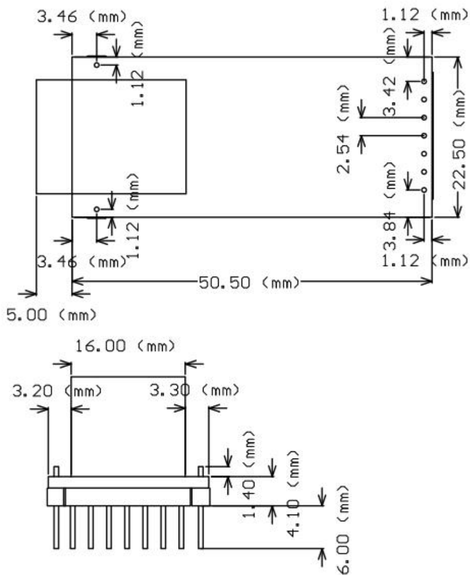
图 5 ZLSN3003S 机械图
